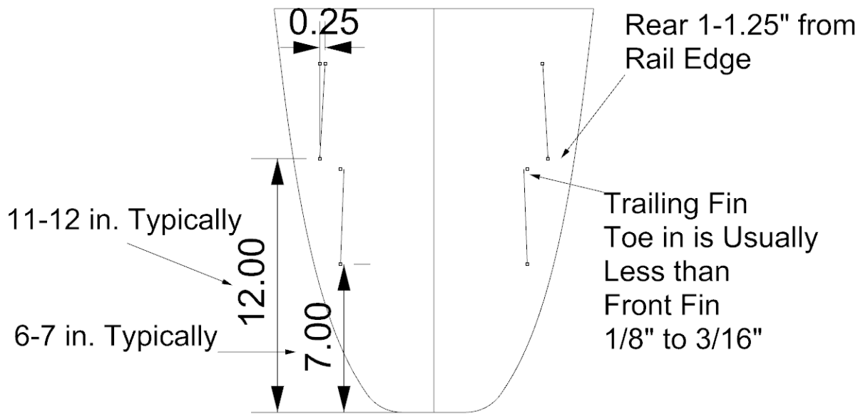
Quad Fin Setup
